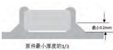
A.回流焊接的最佳焊料用量
