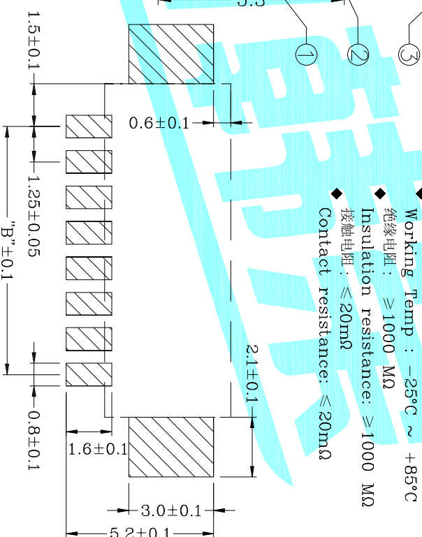
P.C.B Layout
