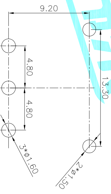
P.C.B layout
