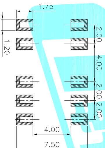
P.C.B layout
