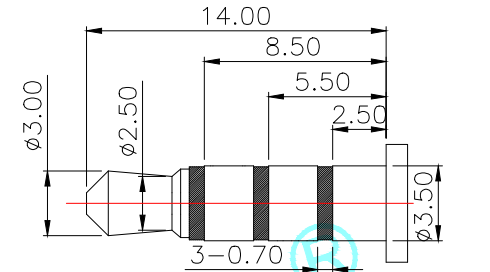
( \phi 3.50\text{mm} 4 POLE PLUG )
