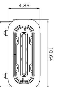
加防水圈示意图
