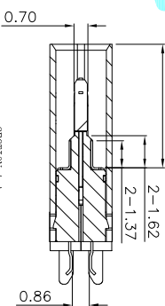
SECTION A-A SCALE 1:1
