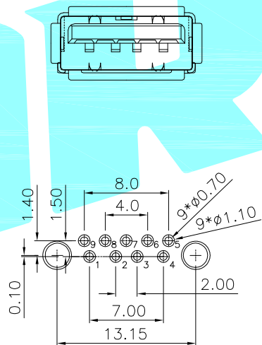
P.C.B LAYOUT TOL: ±0.05
