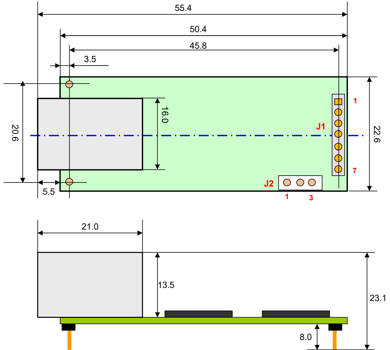
图 2.3 HS-ENG093B 尺寸图
