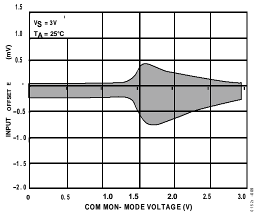
图9. 输入失调电压与共模电压的关系
