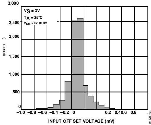
图5. 输入失调电压分布图
