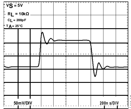
图45. 小信号瞬态响应
