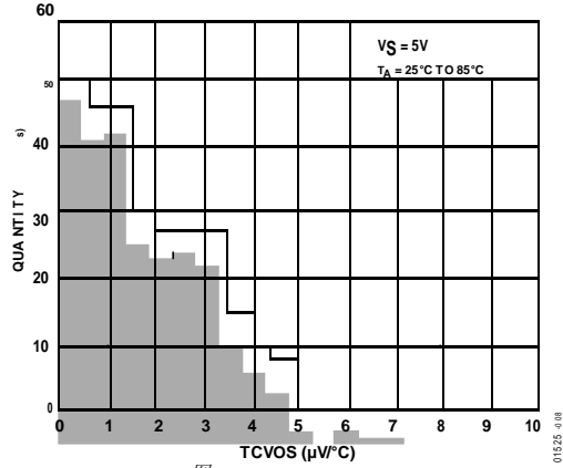
图8. 输入失调电压漂移分布图
