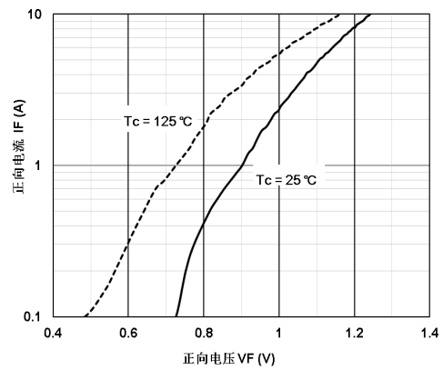
图 12. 二极管的正向压降特性
