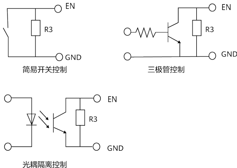
图 6-4 EN 引脚控制方式推荐图
