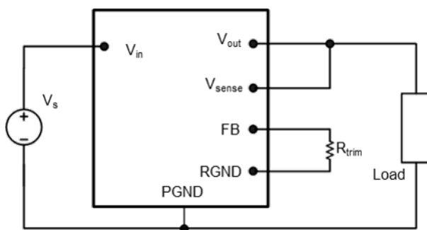
图 6-6 R trim 外部连接
