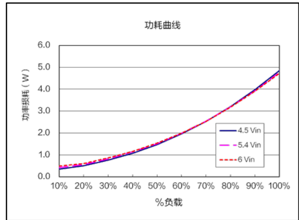
功耗曲线 ( V_{nom}=5.4V , V_{out}=1.8V )
