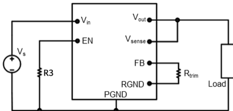
图 6-5 EN 功能电路配置图
