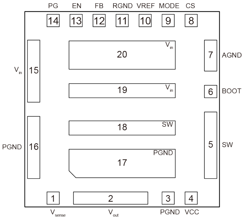
图 6-3 引脚分布
