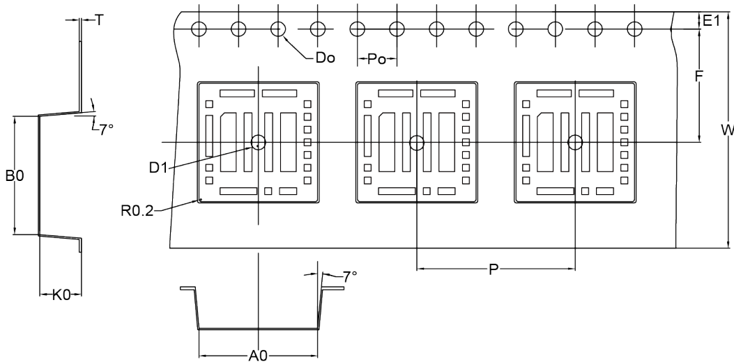
图 12-2 卷带尺寸
