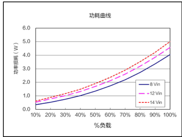
功耗曲线 ( V_{nom}=12.0V , V_{out}=1.0V )
