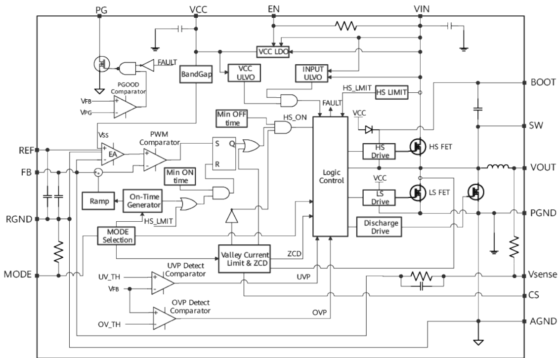
图 3-1 原理框图
