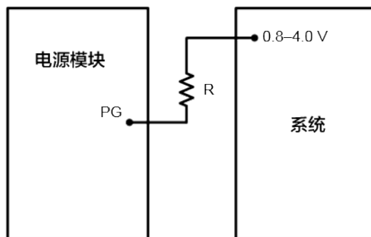
图 6-7 PG 配置图
