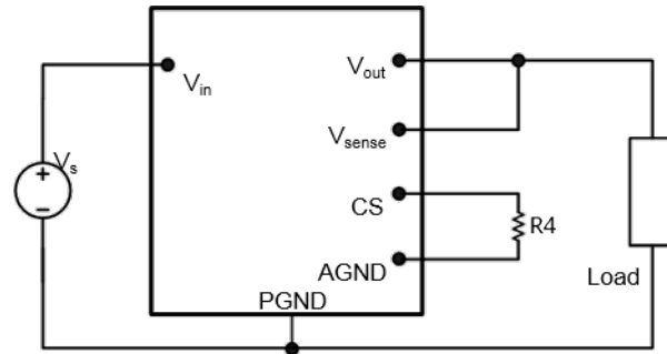
图 6-8 限流电阻外部连接
