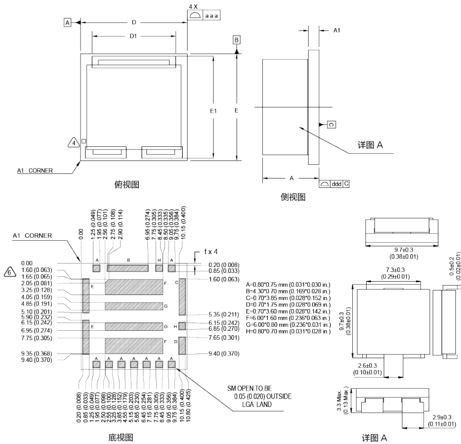
图 6-2 结构尺寸图
