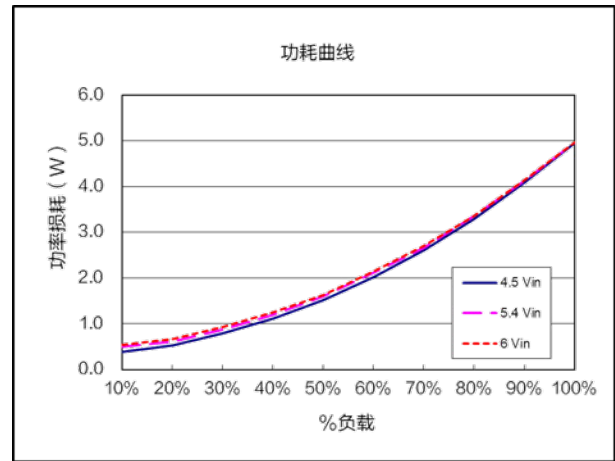
功耗曲线 ( V_{nom}=5.4V , V_{out}=2.1V )
