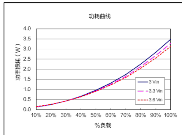
功耗曲线 ( V_{nom}=3.3V , V_{out}=0.6V )
