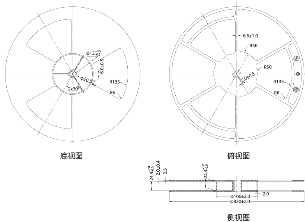
图 12-1 卷盘尺寸
