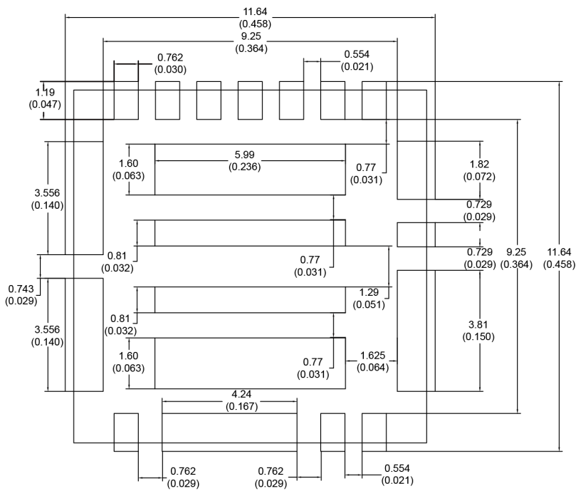
图 6-1 封装尺寸图
