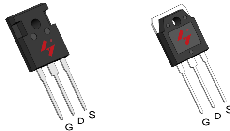
TO-247A-3L
