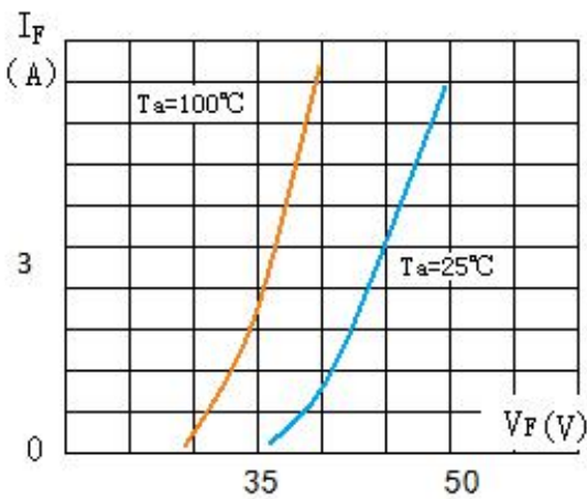
正向特性曲 ( 2CL35KV/3A ) Forward Characteristics
