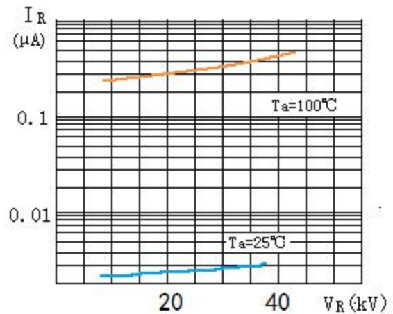
反向特性曲线 ( 2CL35KV/3A ) Reverse Characteristics
