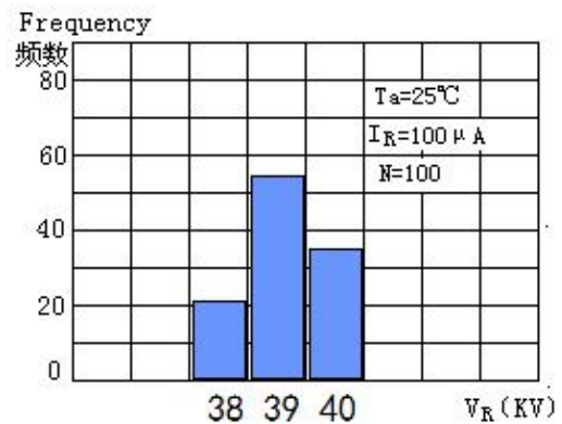
反向雪崩电压分布 ( ( 2CL35KV/3A ) Avalanche Breakdown Voltage Distribution
