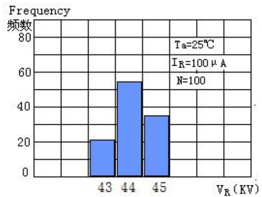
反向雪崩电压分布 ( 2CL40KV/3A ) Avalanche Breakdown Voltage Distribution
