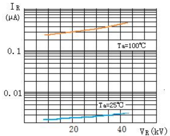
反向特性曲线 ( 2CL40KV/3A ) Reverse Characteristics
