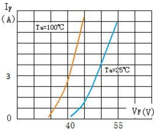
正向特性曲 ( 2CL40KV/3A ) Forward Characteristics
