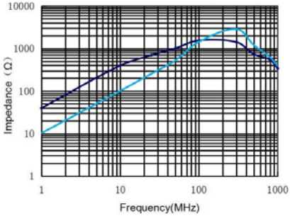
CMF9070-301-2P-T
