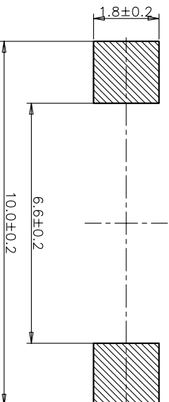
RECOMMENDED P.C.B. LAYOUT 安装尺寸图
