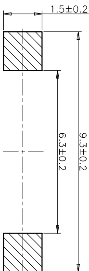
RECOMMENDED P.C.B. LAYOUT 安装尺寸图
