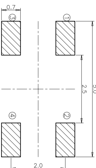
RECOMMENDED P.C.B. LAYOUT 安装尺寸图
