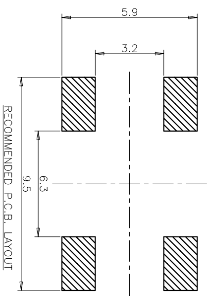
安装尺寸图
