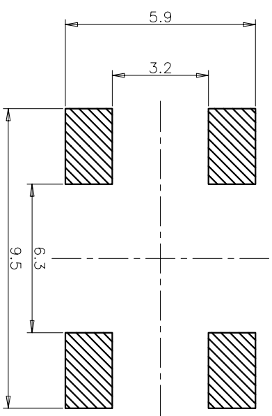
RECOMMENDED P.C.B. LAYOUT 安装尺寸图
