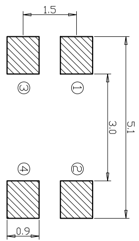
RECOMMENDED PCB LAYOUT 安装尺寸图
