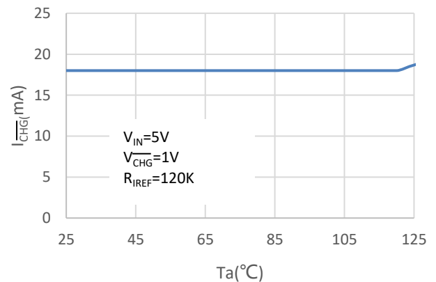
I_{CHG} vs T_a
