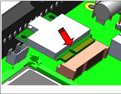
Fig. 8-1 Insert Half-sized Mini PCI-e module
