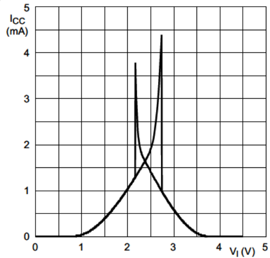
图9 典型AiP74AHC1G14传输特性; V_{CC}=4.5V
