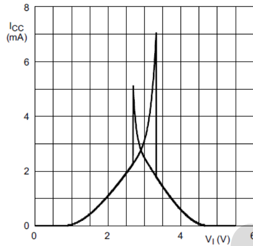
图10 典型AiP74AHC1G14传输特性; V_{CC}=5.5V
