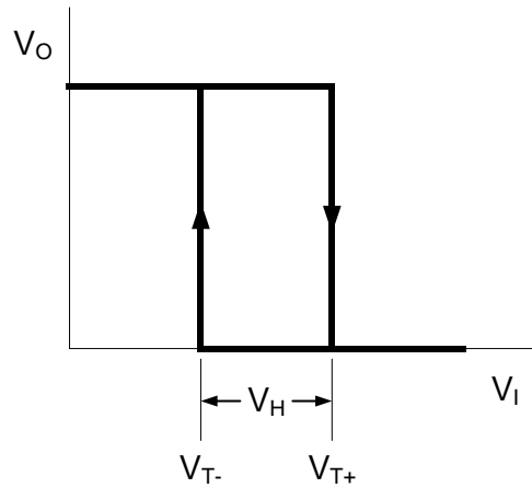
图6 传输特性
