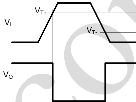
图7 V_{T+} , V_{T-} 和 V_H 的定义
