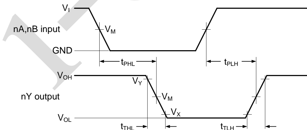
图5 输入到输出传输延迟及输出转换时间
