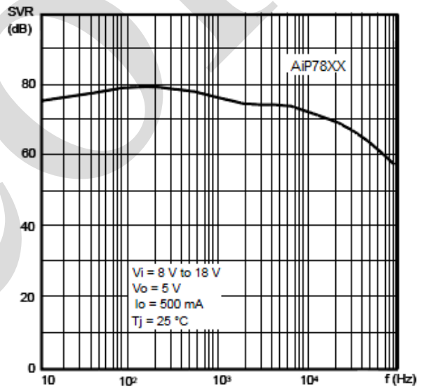
纹波抑制比
