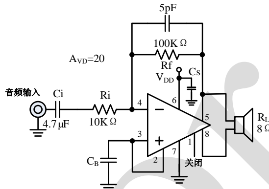
图3、高增益电路
