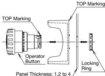
ø22 mm
