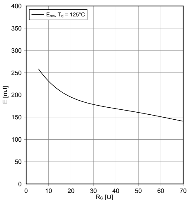
Schaltverluste Diode, Wechselrichter (typisch) switching losses Diode, Inverter (typical) E_{rec} = f(R_G)
