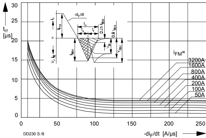
Bild / Fig. 4 Sperrverzögerungszeit t_{rr} (Richtwert für obere Streubereichsgrenze) in Abhängigkeit von der abkummierenden Stromsteilheit bei t_{vj} = 150^\circ\text{C} , V_R = 100\text{V} , V_{RM} \leq 200\text{V} . Parameter: Durchlaßstrom vor der Kommutierung.
