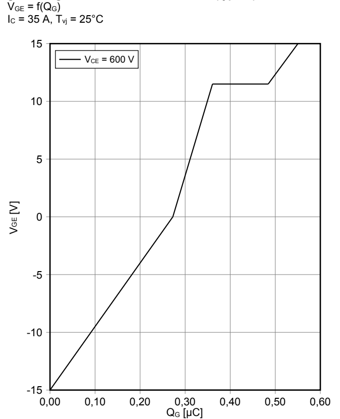
Gateladungs Charakteristik IGBT, Wechselrichter (typisch) gate charge characteristic IGBT, Inverter (typical) V_{GE} = f(Q_G) I_C = 35\text{ A} , T_{vj} = 25^\circ\text{C}
