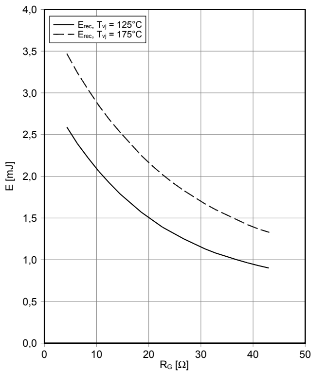
Schaltverluste Diode, Wechselrichter (typisch) switching losses Diode, Inverter (typical) E_{rec} = f(R_G) I_F = 50 A, V_{CE} = 600 V
