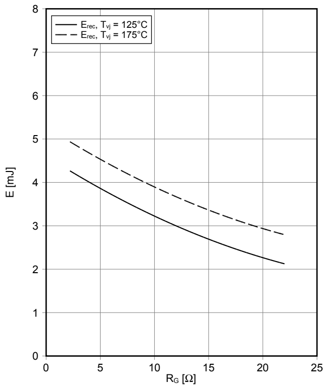
スイッチング損失 Diode、インバータ (Typical) switching losses Diode, Inverter ( typical ) E_{rec} = f(R_G) I_F = 75 A, V_{CE} = 600 V
