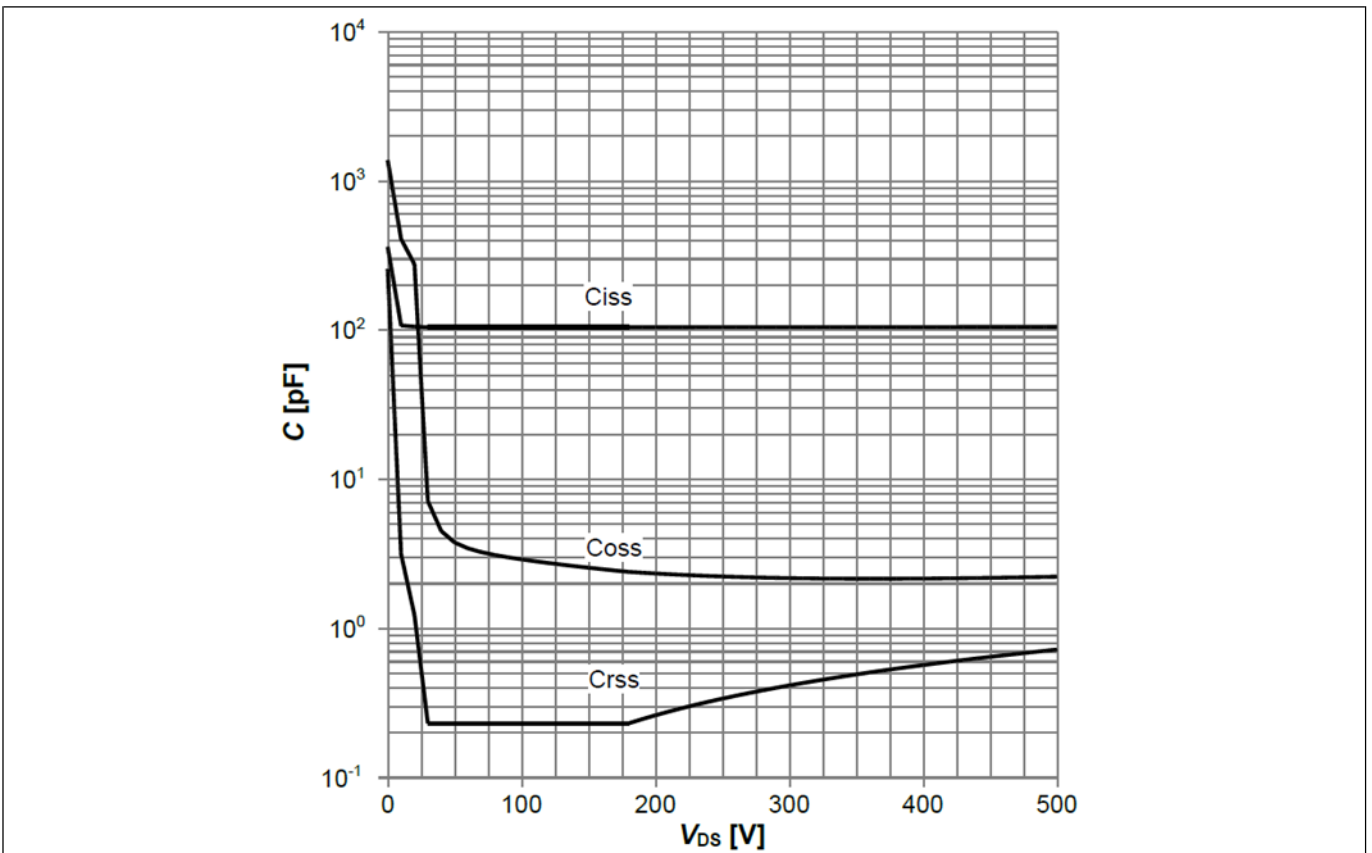
图 23 ICE5QR4780BG 的典型 CoolMOS™ 电容 ( C=f(V_{DS}) ; V_{GS}=0\text{ V} ; f=250\text{ kHz} )
