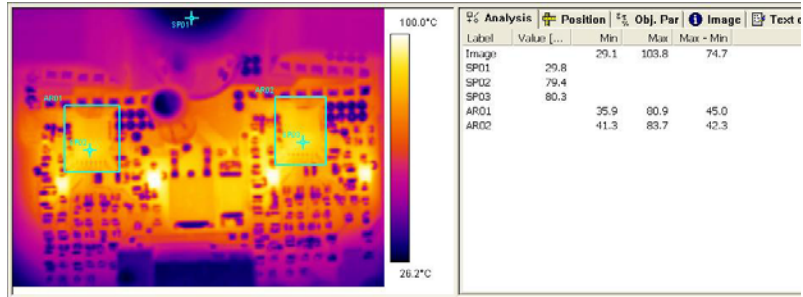
Fig 7 IRAUDAMP15 (Vbus=31V)
