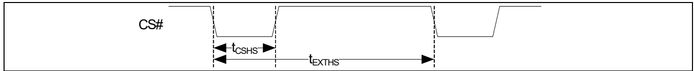
Figure 16 HS トランザクション終了
