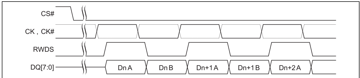
Figure 7 読み出しトランザクション中のデータ配置 [12,13,14,15,16]
