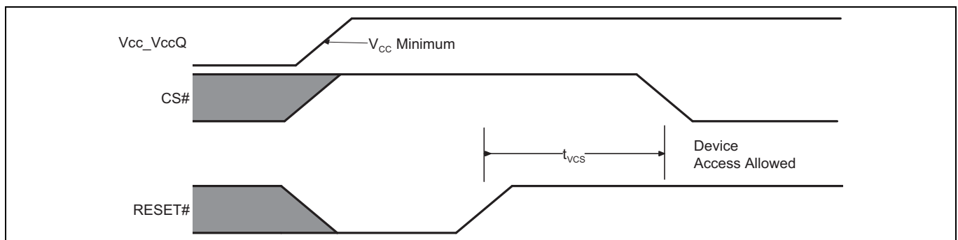
Figure 22 RESET# が LOW 時の電源投入
