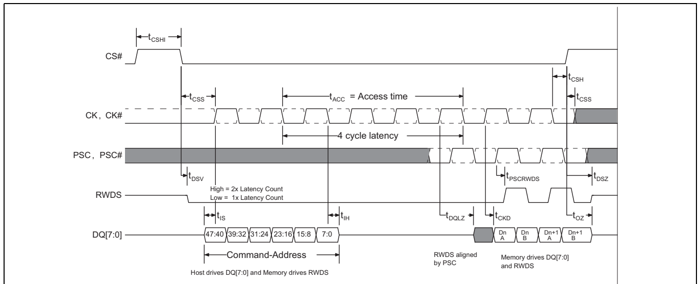
Figure 39 HYPERRAM™ メモリの DCARS タイミング図 [70,71,72]
