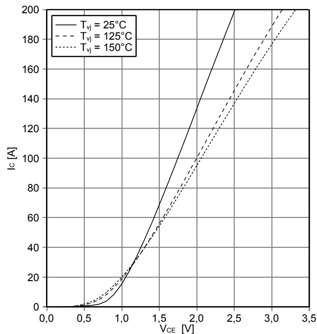
Ausgangskennlinie IGBT, Brems-Chopper (typisch) output characteristic IGBT, Brake-Chopper (typical) I_C = f(V_{CE}) V_{GE} = 15\text{ V}
