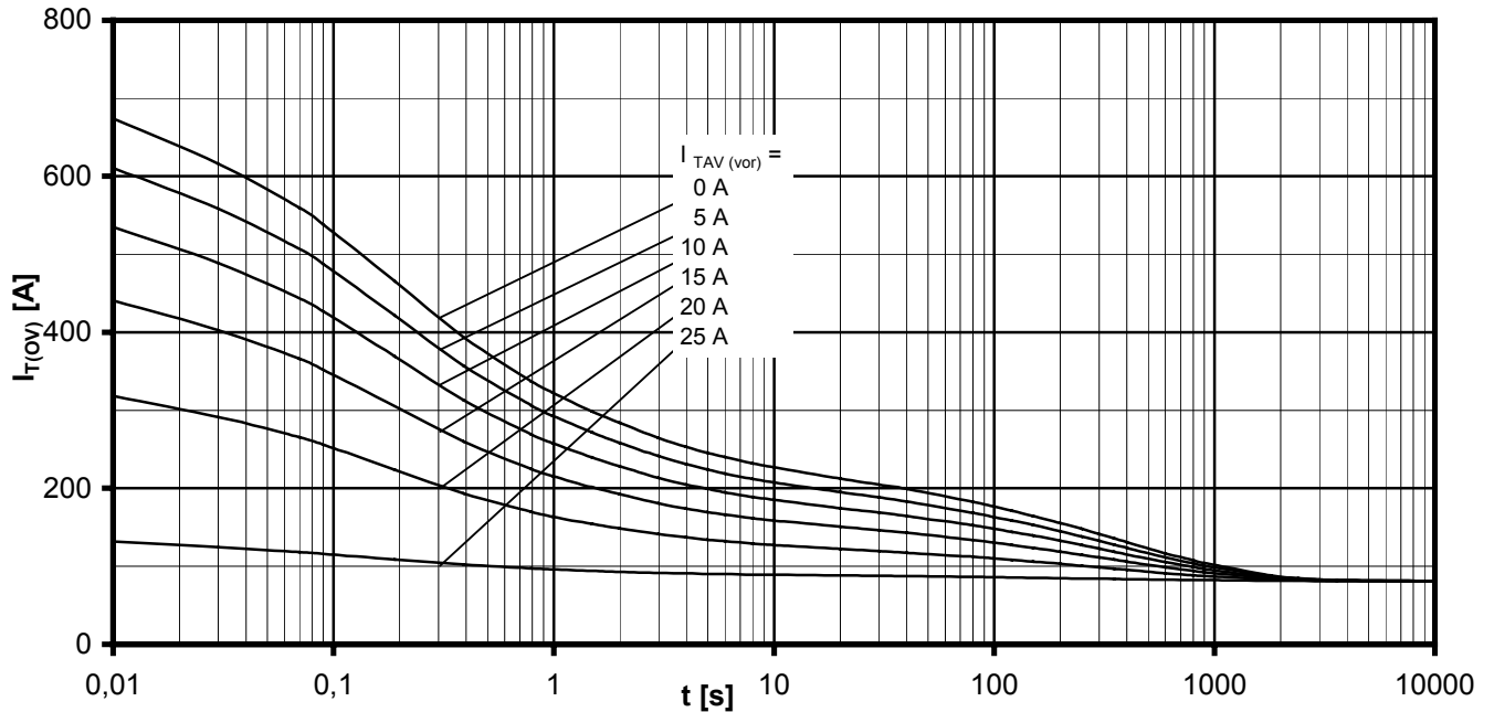
Überstrom je Zweig / Overload on-state current I_{F(ov)}
