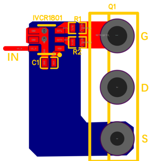
IVCR1801 布局实例
