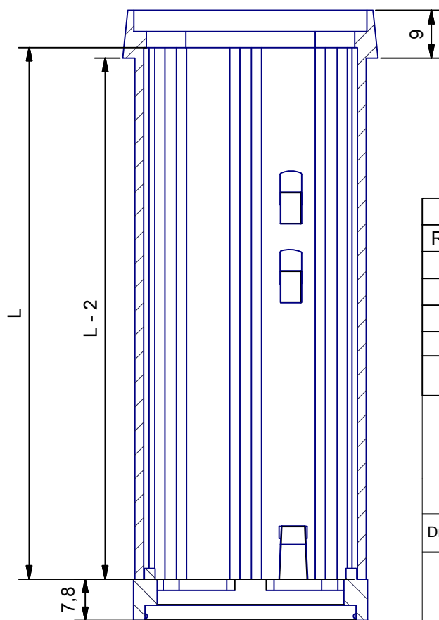
A-A (1:1)
