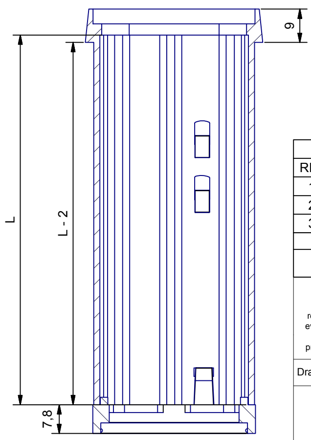
A-A (1:1)
