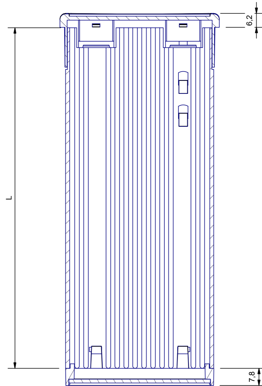
A-A (1:1)
