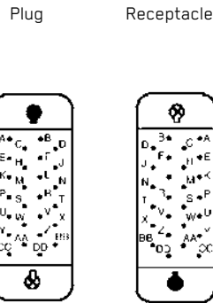
50-way
