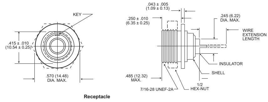
Receptacle
