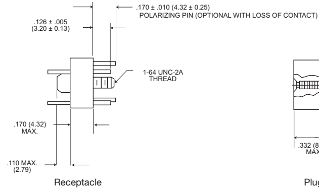
Receptacle
