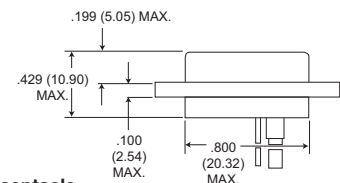
Receptacle
