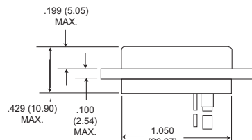
Receptacle
