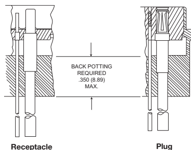
Receptacle
