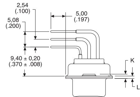
DD Configuration
