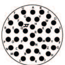
25-37 - 25-37* 37 #16 I
