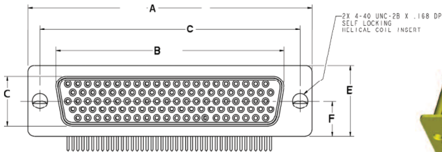
Receptacle - Socket
