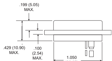
Receptacle
