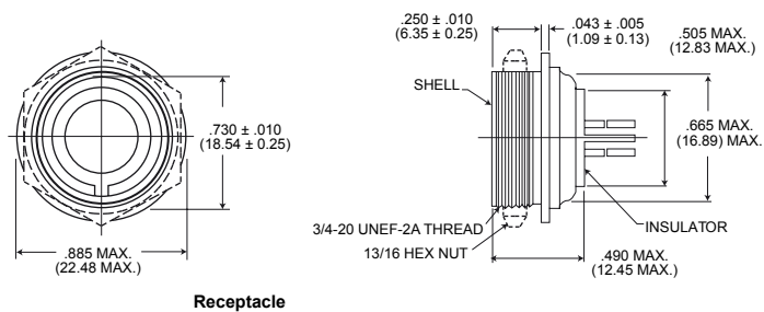
Receptacle
