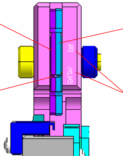
芯線クリンパ Wire Crimper
