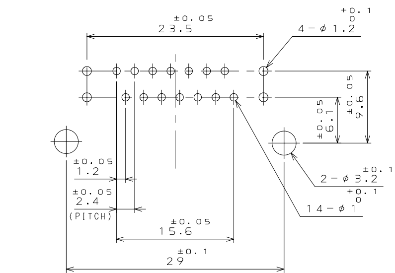
P.C.B. HOLE PATTERNS (REF.) 基板取付穴寸法 (参考) THICKNESS (基板厚): t 1.6 ±0.2
